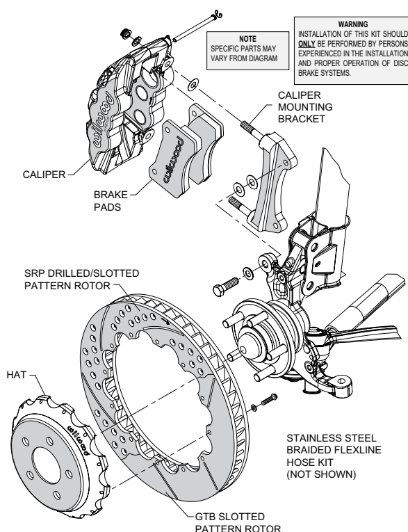
AERO6 Front, Spec37 GTB Slotted Rotor
